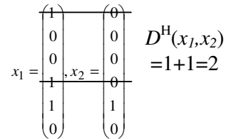
Рис. 7б. Расстояние Хэмминга
