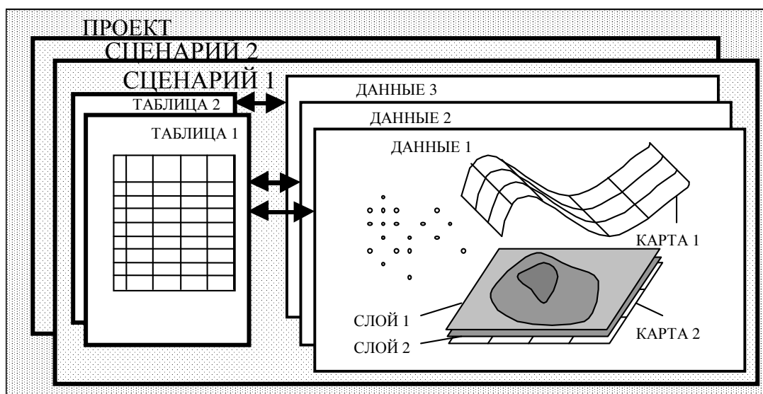
Рис.37. Внутренняя структура объектов программы ViDa Expert
