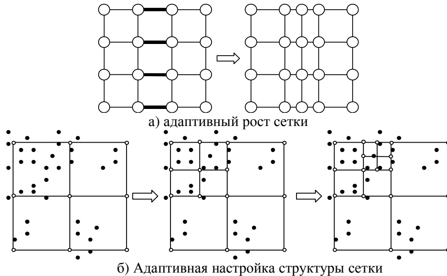
Рис. 33. Иллюстрации к работе алгоритмов адаптивного изменения структуры сетки
