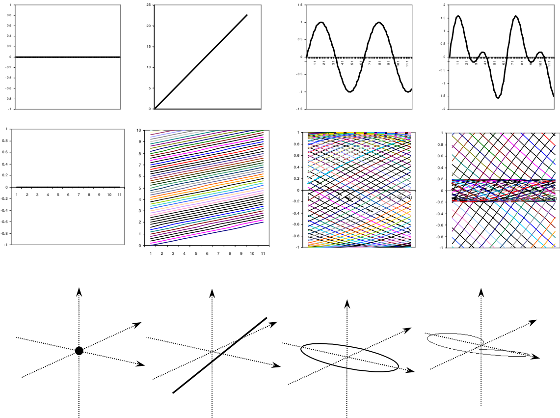
Рис.34. Иллюстрации к вложению временных рядов по Такенсу
